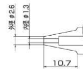
N3-13 Nozzle Size \Phi 1.3
