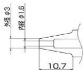
N3-16 Nozzle Size \Phi 1.6
