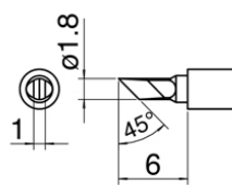
T30-KU Shape-KU
